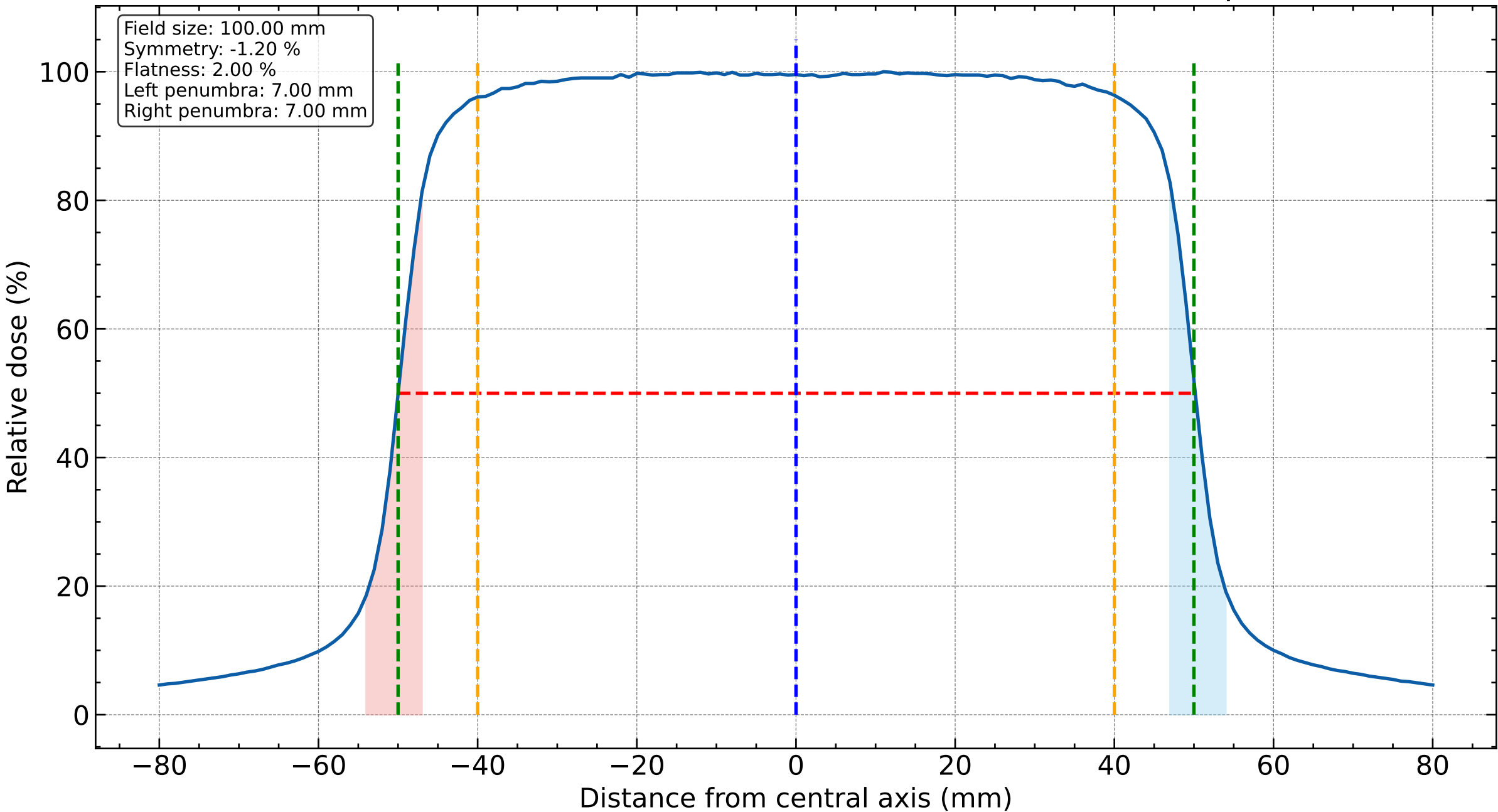
10MV, Beam Profile(Inline), SSD=100CM, F.S=10X10 cm 2 , Depth=10cm
